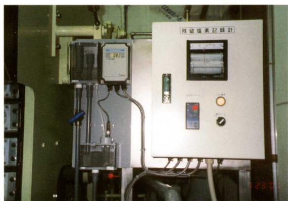
▲高濃度残留塩素管理ユニット
