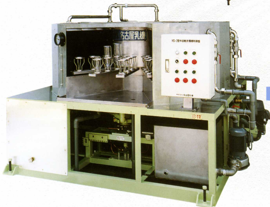
HS-3型ロータリー洗壺機
