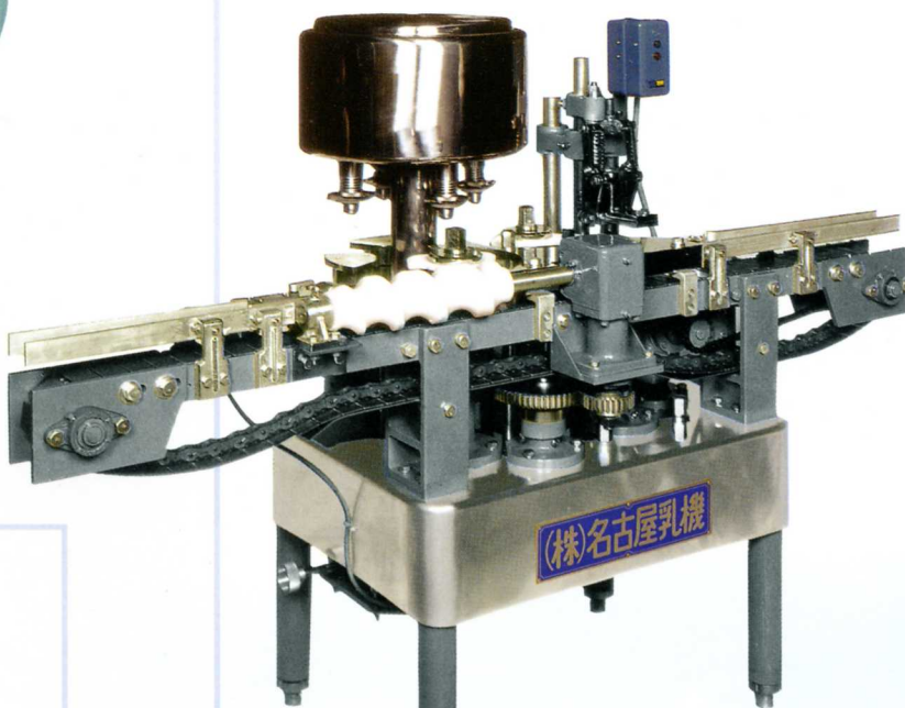
SM4×1型全自動壘詰打栓機
