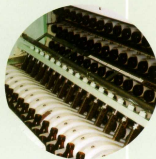
▲NDS16列式全自動洗壺機 給壺部
