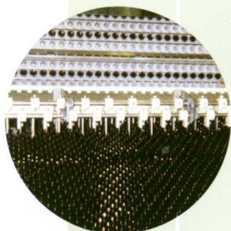
▲NDS30列式全自動洗壺機 給壺部
